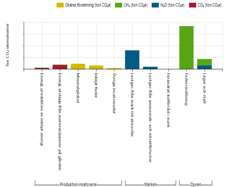
Summering växthusgasutsläpp
