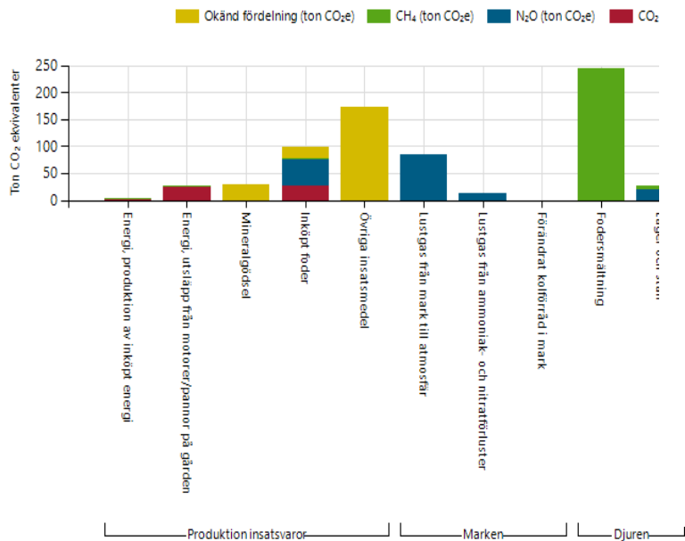
Summering växthusgasutsläpp
