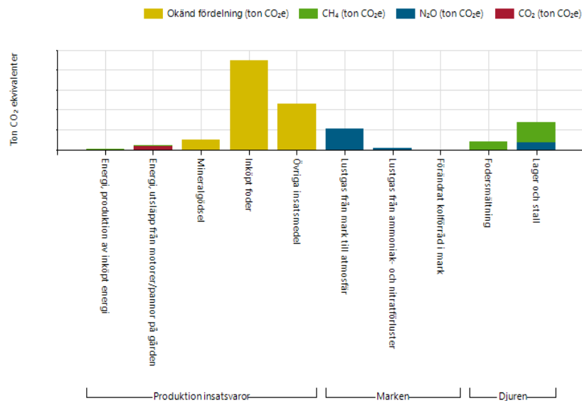
Summering växthusgasutsläpp
