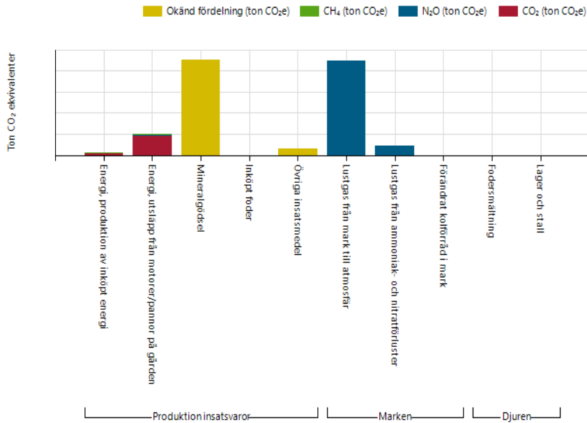
Summering växthusgasutsläpp
