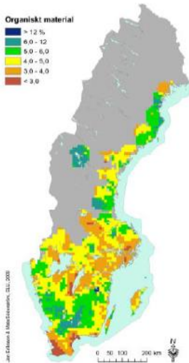
Karta 4. Hält organiskt material i markjorden. Data från omdrev 1 och 2 sammanslagna. Antal värden 5 179. Map 4. Organic matter content in the topsoil. Data from sampling series 1 and 2 combined (n = 5 179).
